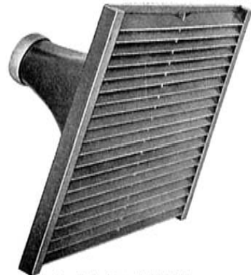
Abb. 4. Akustische Linse, Vorderseite
